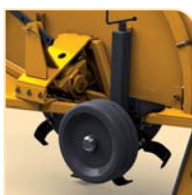
Ruota regolazione profondità Depth adjustment wheel
